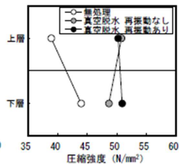
図14 圧縮強度分布
