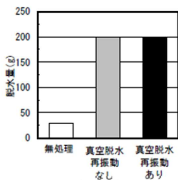
図12 脱水量
