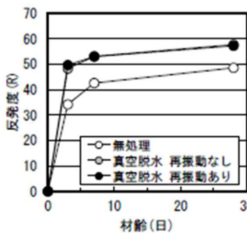
図13 材齢と反発度
